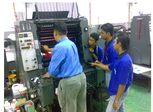
Latihan mencetak mesin M-Offset
